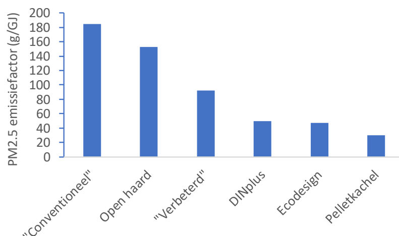
Figuur 1 PM 2.5 emissiefactoren per type houtkachel (exclusief condenseerbare fractie).
